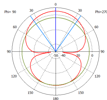
Н-площина(Horwin AD3501)
