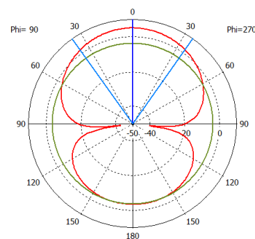
Н-площина (Horwin AD 4501)
