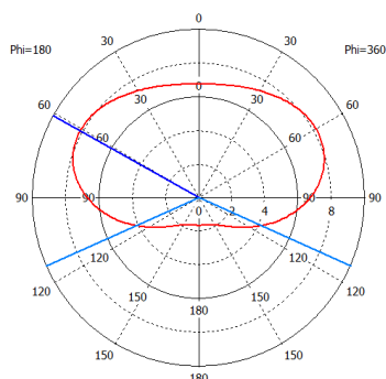
Е-площина 3/8 λ від мачти
