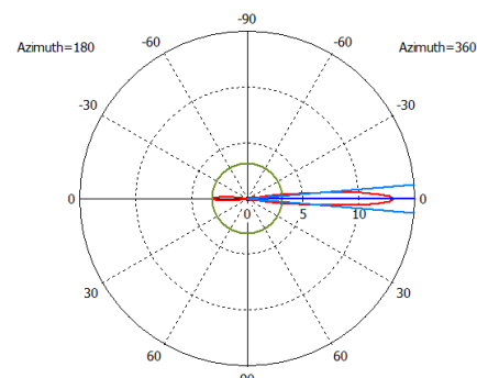
Н-площина (Horwin AD 4508)
