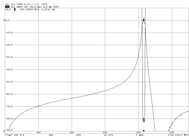
Графік КСХ
