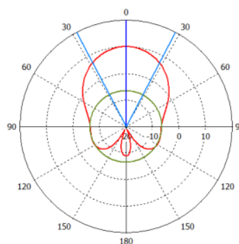
Н-площина (Horwin AP1800)
