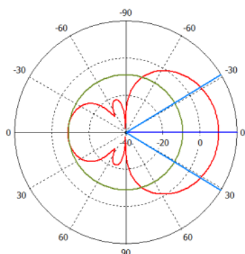
Е-площина (Horwin AP1800)
